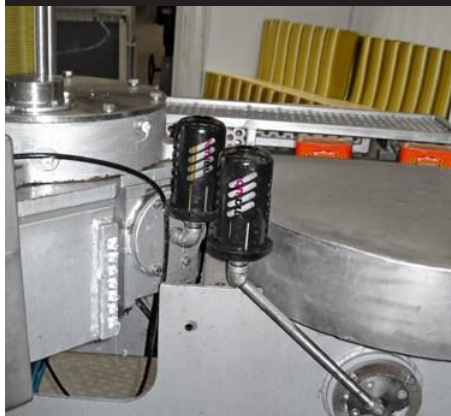
상승부 컨베이어의 구동 장치에 있는 플랜지 베어링의 윤활
